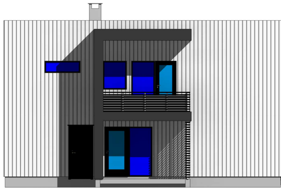
Fasade Nord 1 : 100
