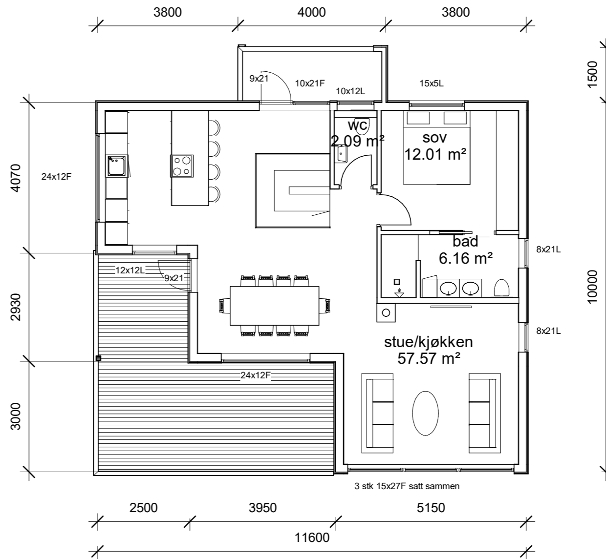
Plan 02 1 : 100
