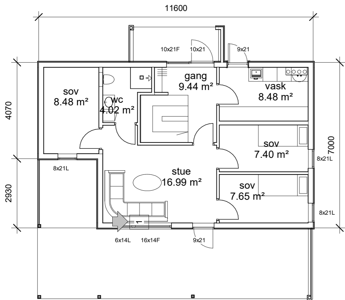
Plan 01 1 : 100
